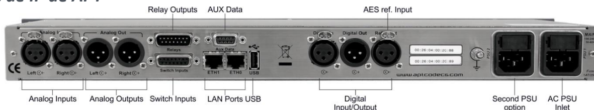
Figura 31: muestra los componentes del panel posterior del códec IP estándar
