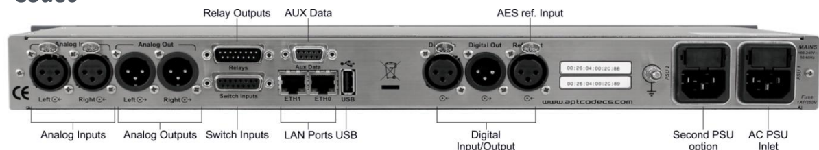
Figure 20 : Composants de la face arrière d'un codec standard
