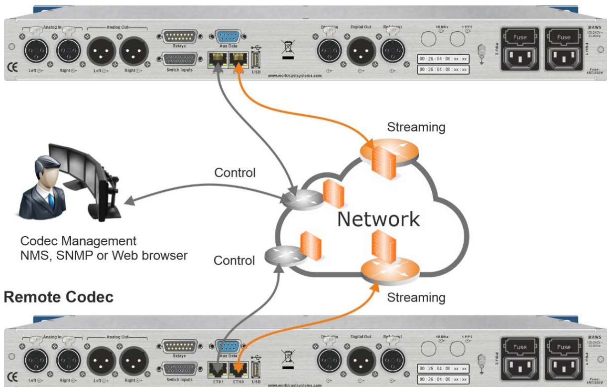
Figure 22: Principe de l'installation du codec dans un réseau générique (APT IP Codec standards)
